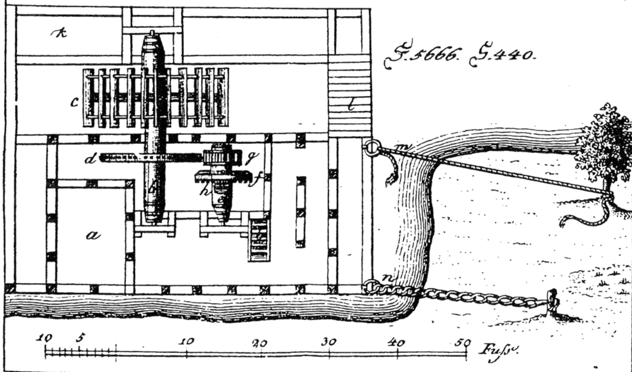
Zeichnung einer gebräuchlichen Schiffmühle mit einem Gang (aus: J.G. Krünitz, Oeconomisch-technologische Encyclopädie, Bd. 95, Taf. 34)
